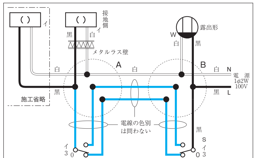
複線結線参考図
