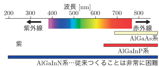
第7図 各化合物半導体材料 (AlGaInN系, AlGaInP系, AlGaAs系) で実現できる光の波長範囲の概略図
