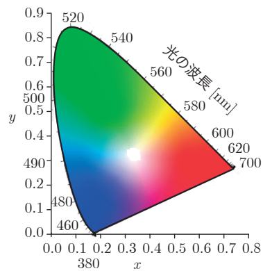
第8図 色度図と光の波長の関係
